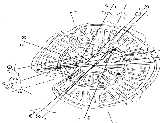
Ил. 4. Аркаим – главни астрономически азимути (схема по изд. „Аркаим : У истоков цивилизации” – 2009)
